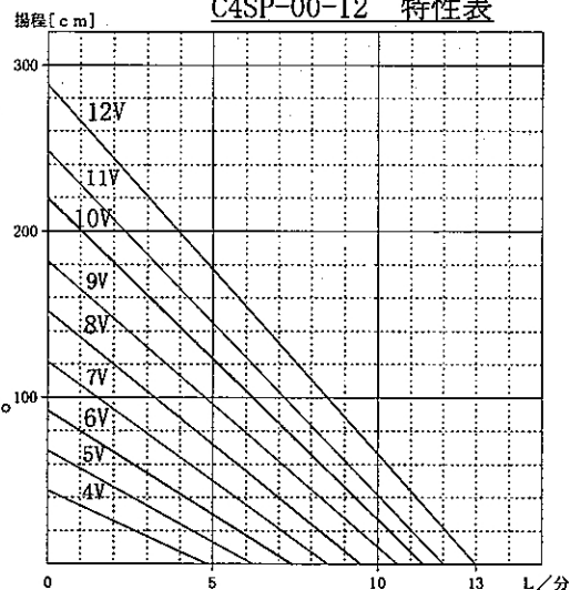
C4SP-00-12 特性表
